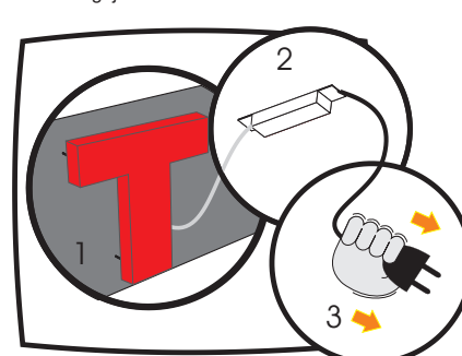
9.- Conectar la última letra al transformador led y éste a la corriente 220V.
