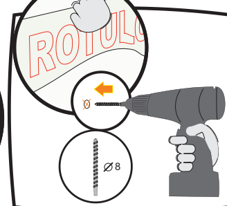
5.- Retirar la plantilla de la pared y realizar un agujero en cada marca de las varillas.
