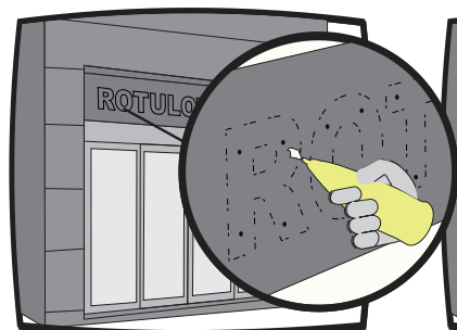
6.- Limpiar el polvo de los agujeros y rellenarlos con cola de montaje. (cola de montaje espesa)
