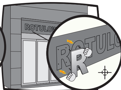
7.- Colocar las letras en sus correspondientes agujeros, moviéndola suavemente hasta que coincida con las marcas de las esquinas.
