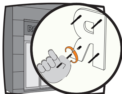
3.- Colocar las varillas atornillándolas en los soportes interiores de las letras. (Podrían entregarse montadas)
