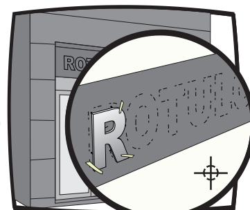
8.- En caso de que se muevan, sujetarlas con cinta de carroceros durante 30 minutos y luego retirar.
